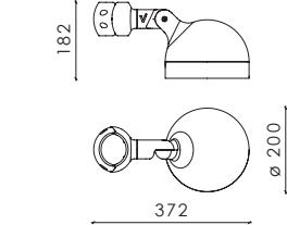
BLACKBIRD MINI SPOT FLANGE MOUNT
