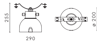
BLACKBIRD MINI HANGING TOOL-LESS
