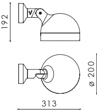
BLACKBIRD MINI FACADE MOUNT
