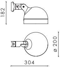
BLACKBIRD MINI SPOT BRACKET MOUNT
