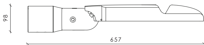
Dimensions avec console réglable ± 90°, 76 mm
