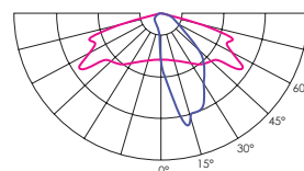
Coupe flux arrière | blanc
